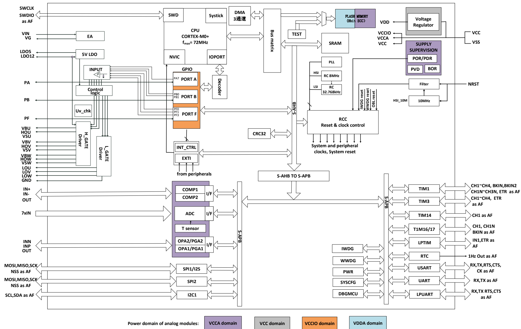
图 1-1 功能模块
