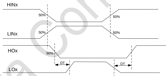
图 5-10 死区功能
