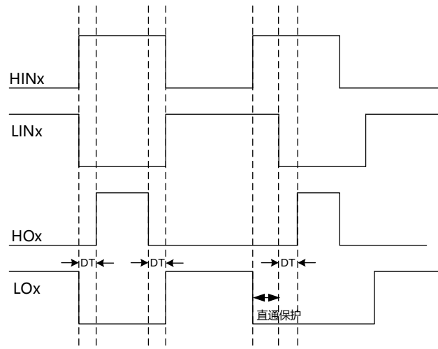
图 5-9 直通保护
