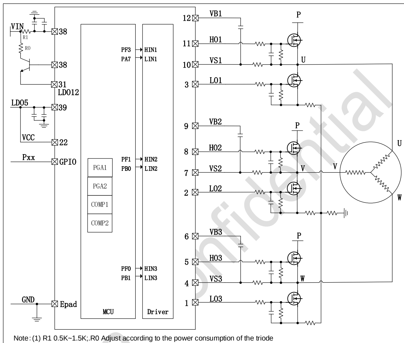
图 6-1 PY32MD530H2 推荐应用电路图
