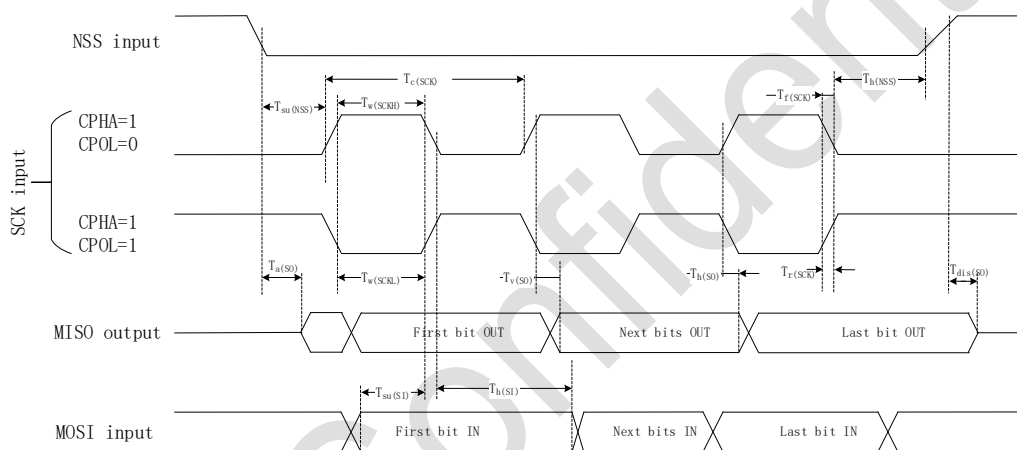
图 5-4 SPI 时序图 – 从机模式, CPHA = 1
