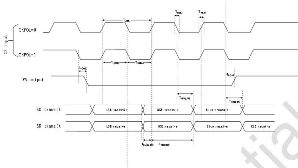
图 5-7 I 2 S 主模式时序图 (Philips 协议)
